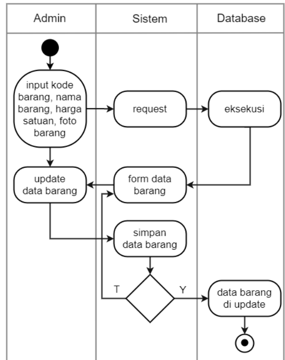
Gambar 6. Mengelola data barang
