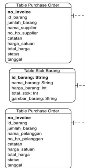
Gambar 7. Desain database
