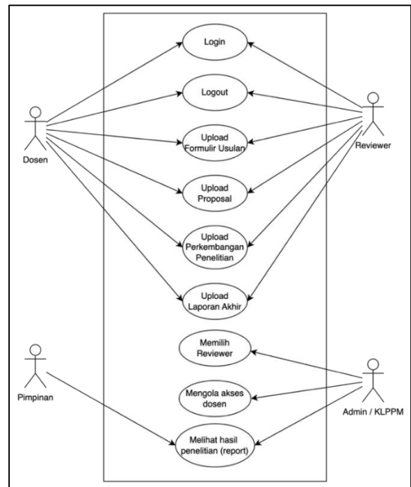
Gambar 2. Use case diagram sistem pengelolaan
