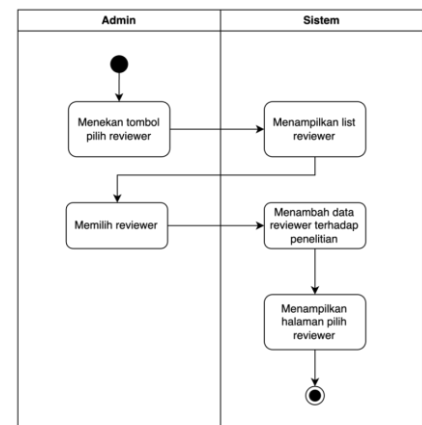
Gambar 6. Activity diagram pemilihan reviewer
