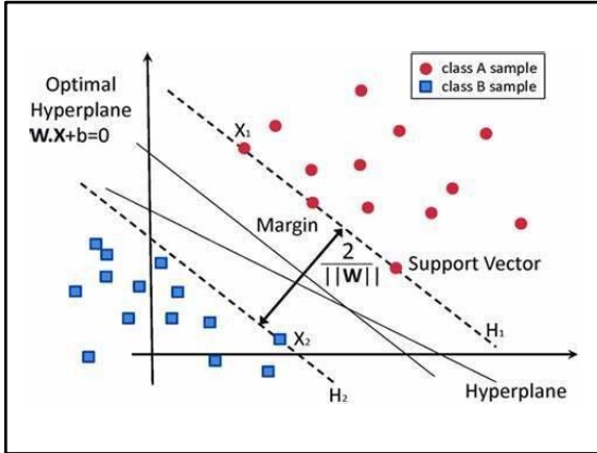
Gambar 1. Klasifikasi Data menggunakan Support Vector Machine (SVM)
