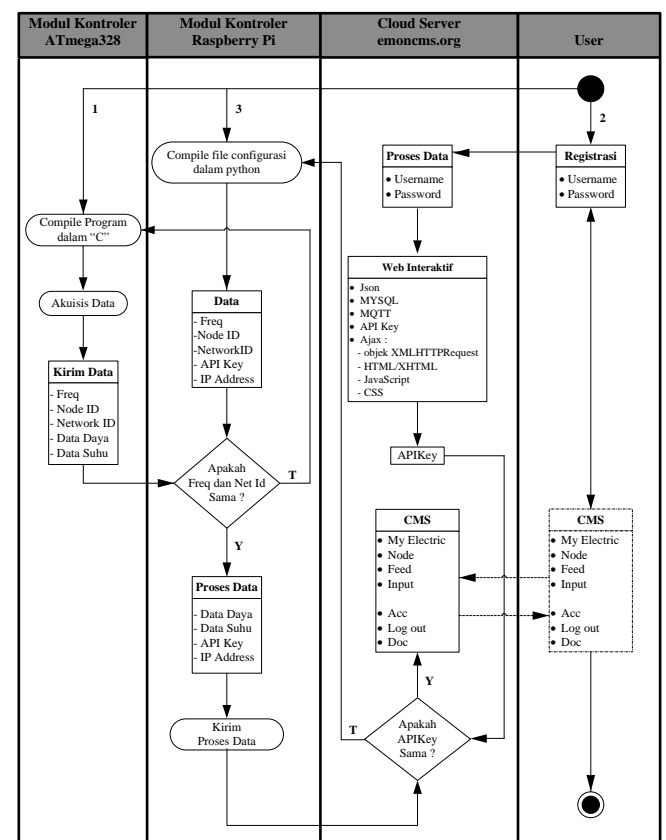
Gambar 3. Perancangan Sistem
