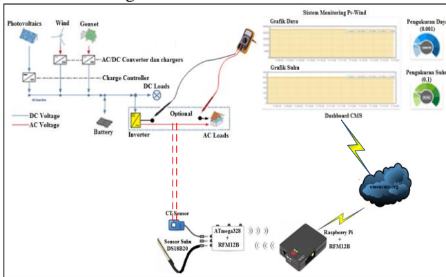
Gambar 2. Arsitektur Sistem Monitoring
