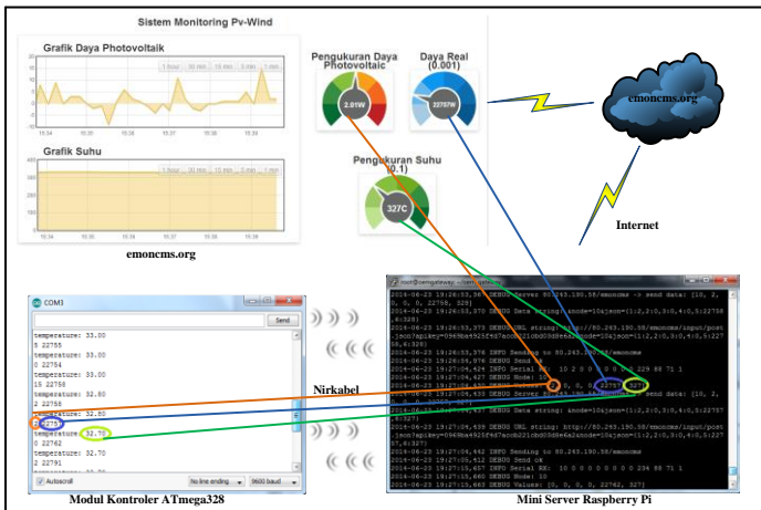
Gambar 4. Proses Aliran Data
